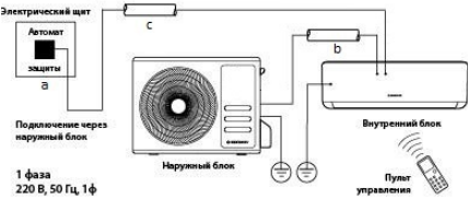
Блок - схема подключения кондиционера к однофазной сети
