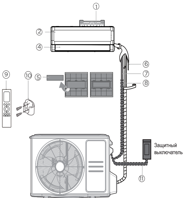
Модели с электропитанием от наружного блока
